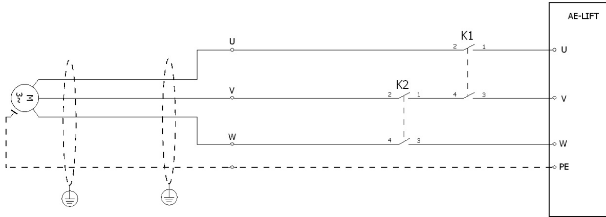
Şekil 4.2 Redüktörlü / Asenkron Motor (Dişlili Makine) Bağlantıları
