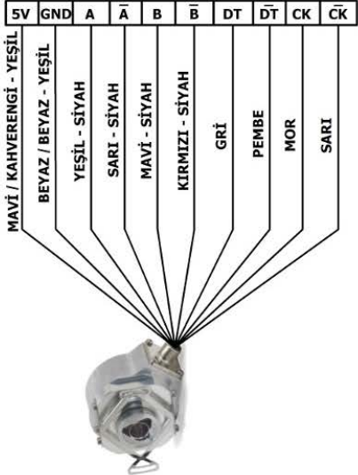
Şekil 4.12 Farklı Mutlak Encoder Modellerine Göre Bağlantı Şekilleri
