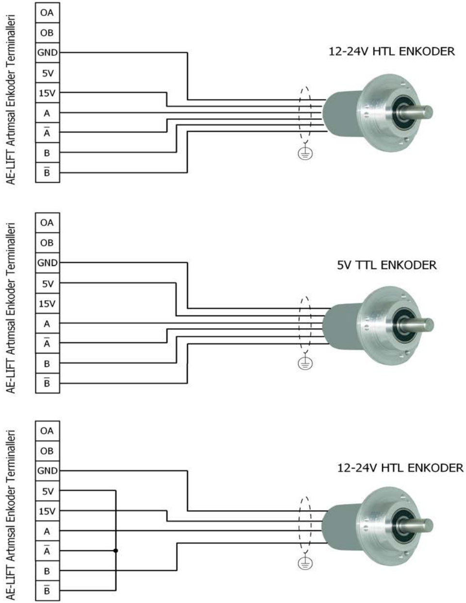
Şekil 4.8 Artımsal Enkoder Bağlantıları
