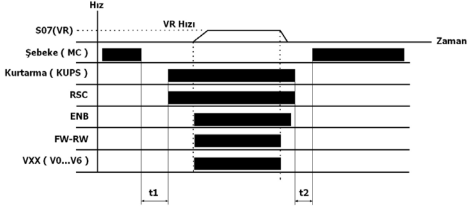
Şekil 8.14 Kurtarıcı Modunda Zamanlar
