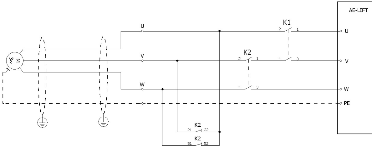
Şekil 4.3 Senkron Motor (Dişlisiz Makine) Bağlantıları
