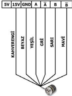
Şekil 4.10 Farklı Artımsal Enkoder Modellerine Göre Bağlantı Şekilleri
