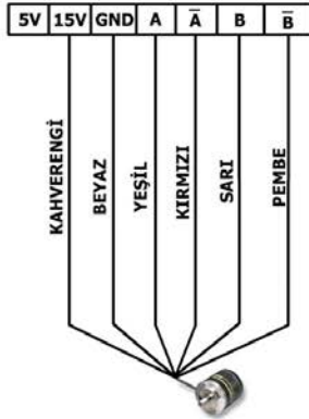
Şekil 4.10 Farklı Artımsal Enkoder Modellerine Göre Bağlantı Şekilleri
