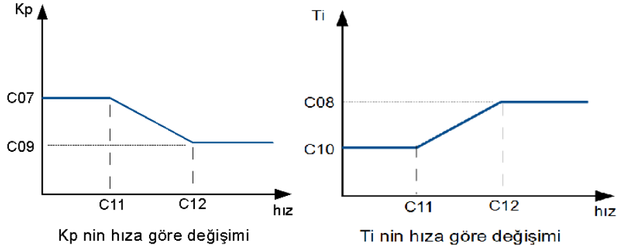
Şekil 8.11 PI Katsayılarının Hıza Göre Değişimi
