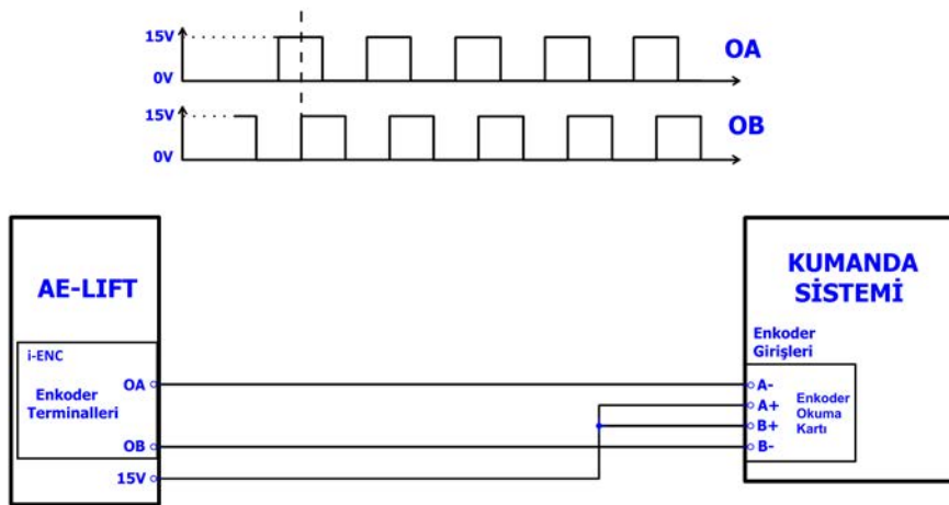
Şekil 4.11 AE-Lift – Kumanda Panosu Enkoder Simülasyon Çıkışı Bağlantıları
